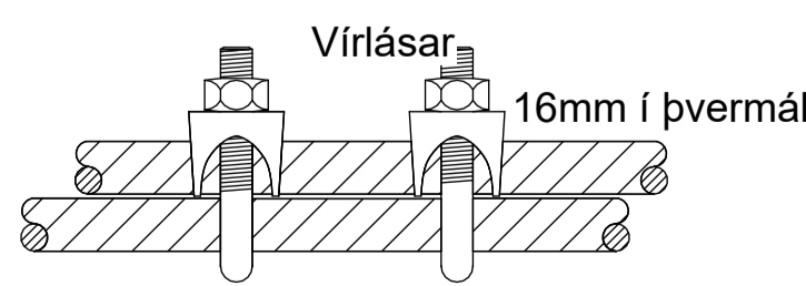
Tveir vírlásar fyrir hver samskeyti
