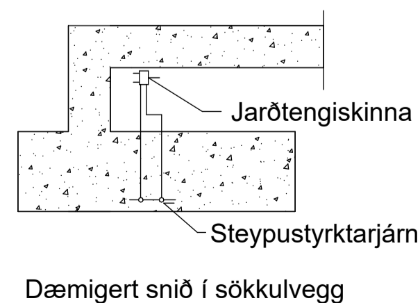
Dæmigert snið í sökkulvegg
