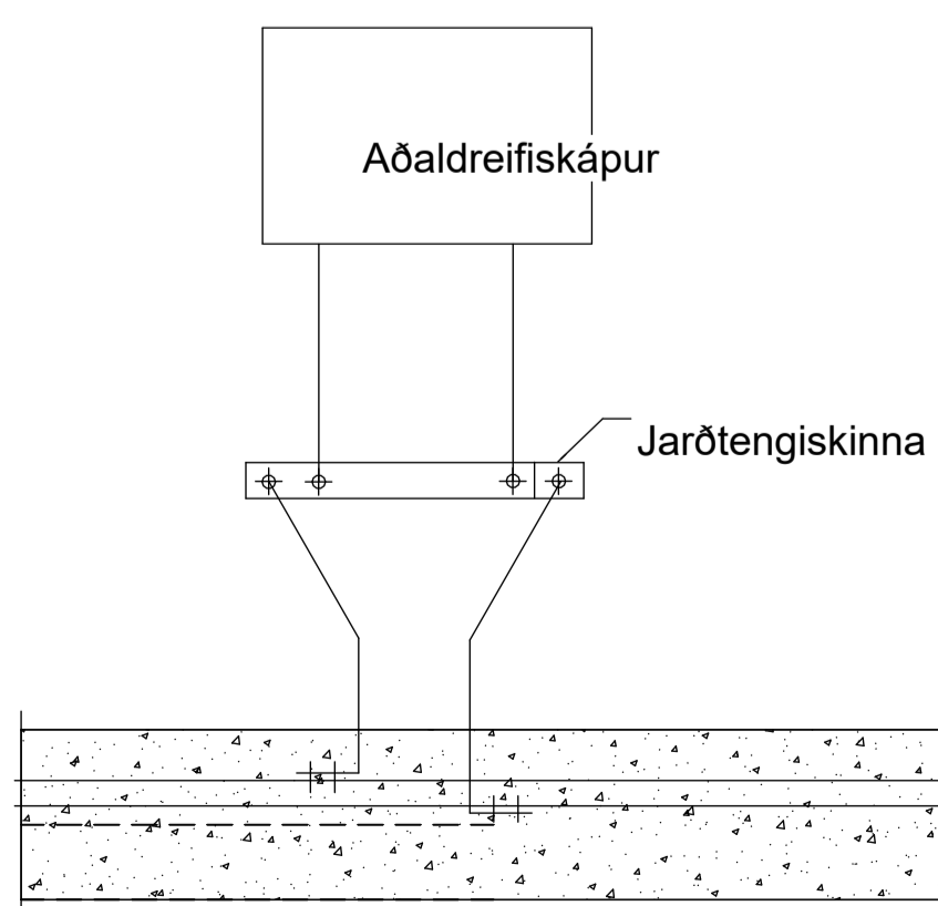
Dæmigerð tenging jarðskauts við jarðtengiskinna
